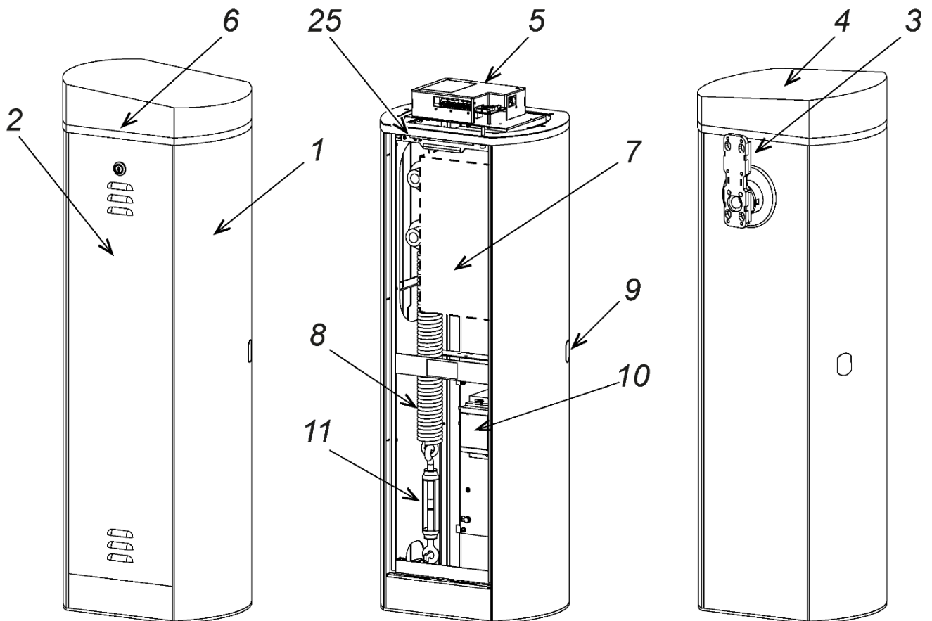
Рисунок 2. Устройство шлагбаума
