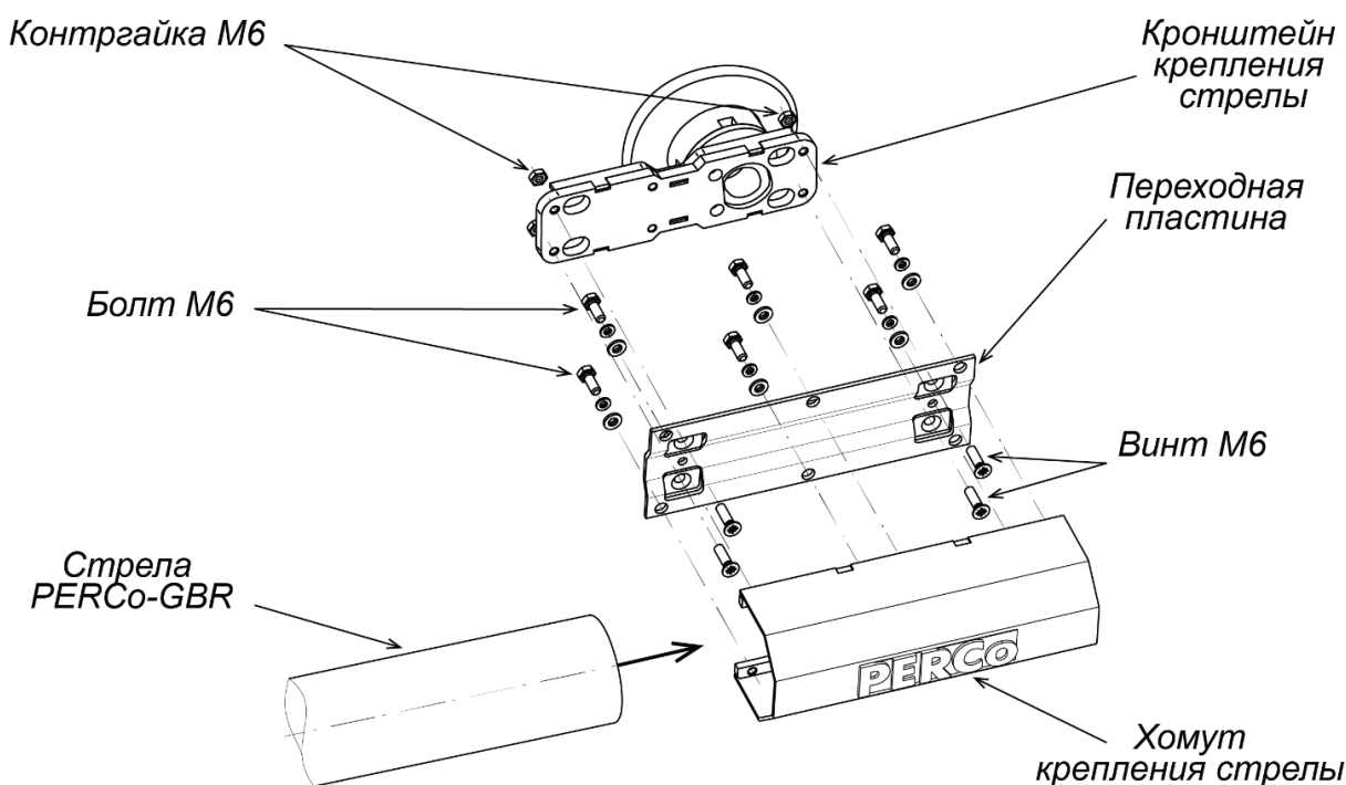
Рисунок 16. Монтаж стрелы PERCo-GBR
