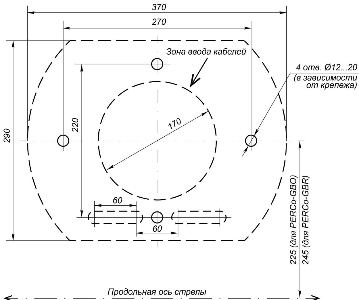
Рисунок 7. Разметка установочных отверстий шлагбаума
