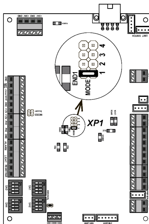
Рисунок 11. Расположение джампера «MODE1» при левостороннем положении стрелы
