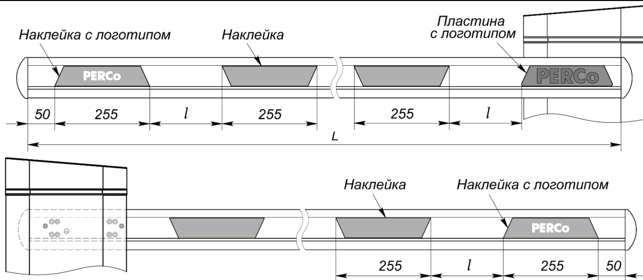
Рисунок 13. Наклеивание световозвращающих элементов на стрелу PERCo-GBO
