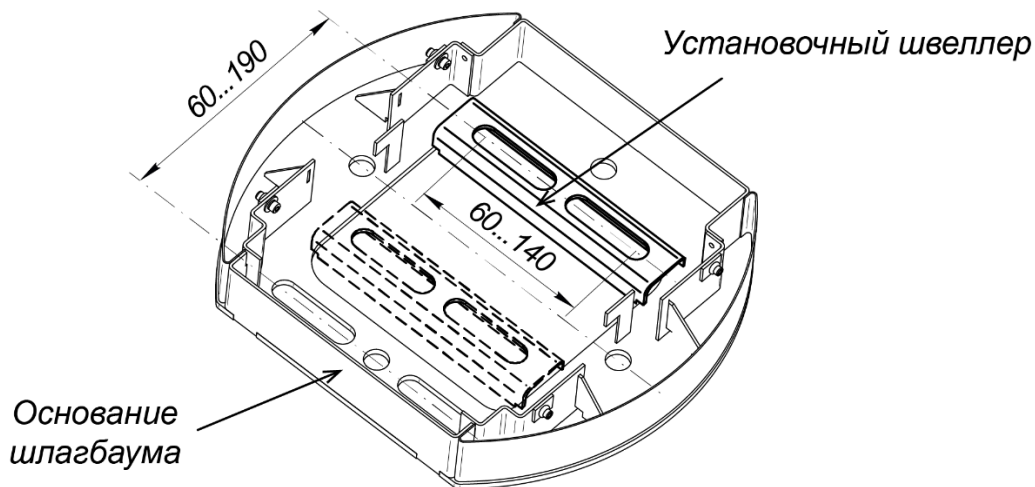
Рисунок 8. Установочный швеллер
