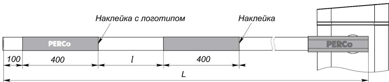
Рисунок 12. Наклеивание световозвращающих элементов на стрелу PERCo-GBR
