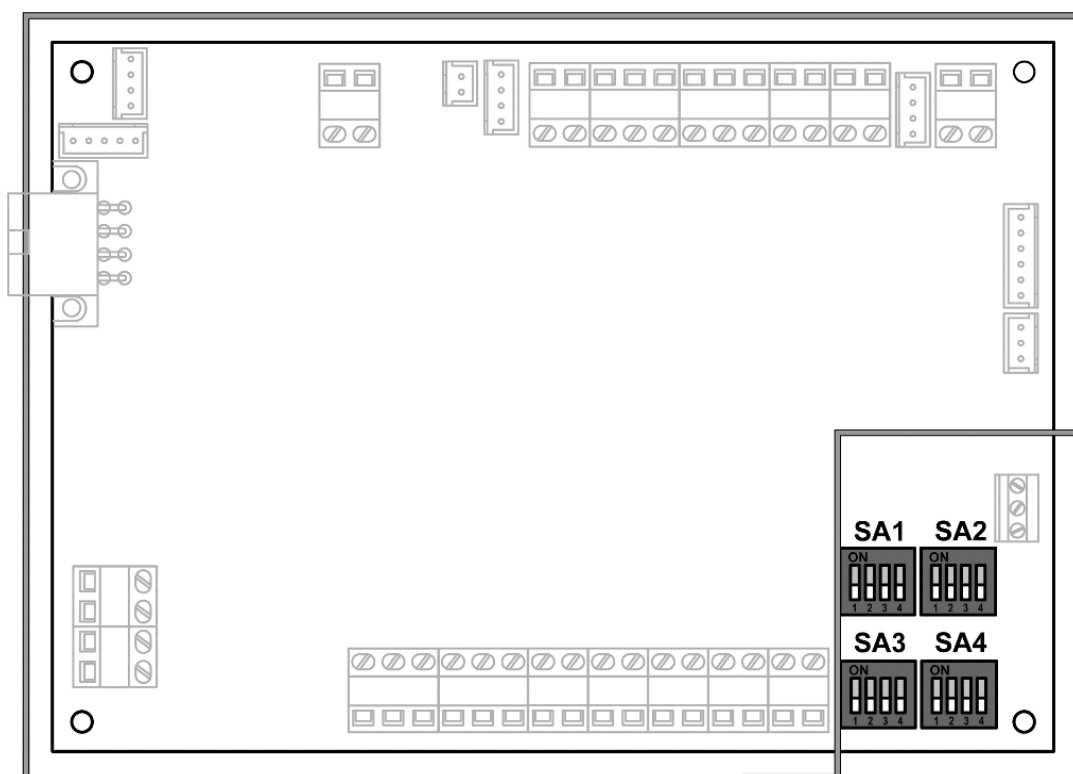
Рисунок 25. Расположение DIP-переключателей на плате управления шлагбаума
