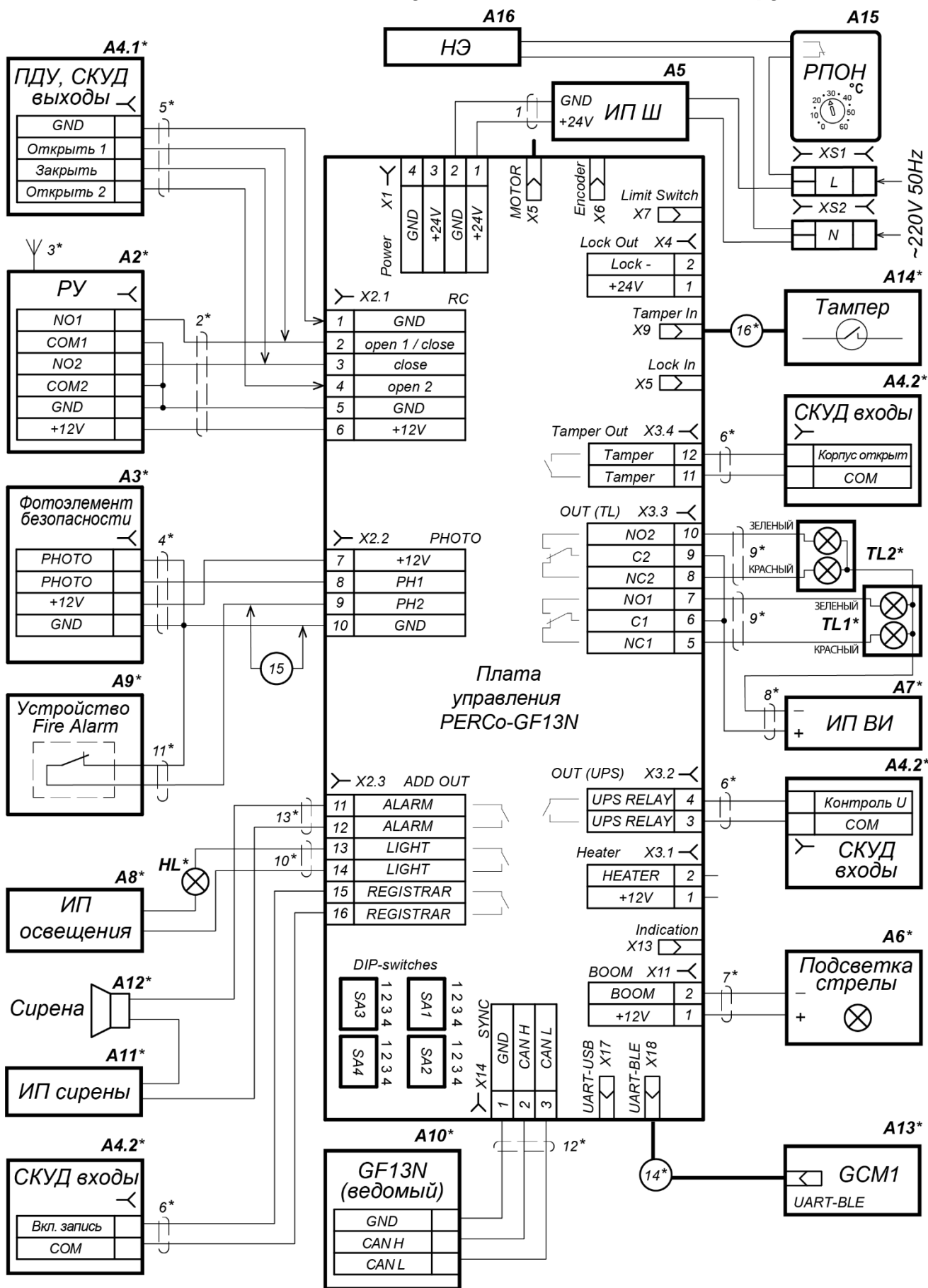
Рисунок 8. Схема подключения шлагбаума и доп. оборудования (перечень элементов см. в табл. 2)
