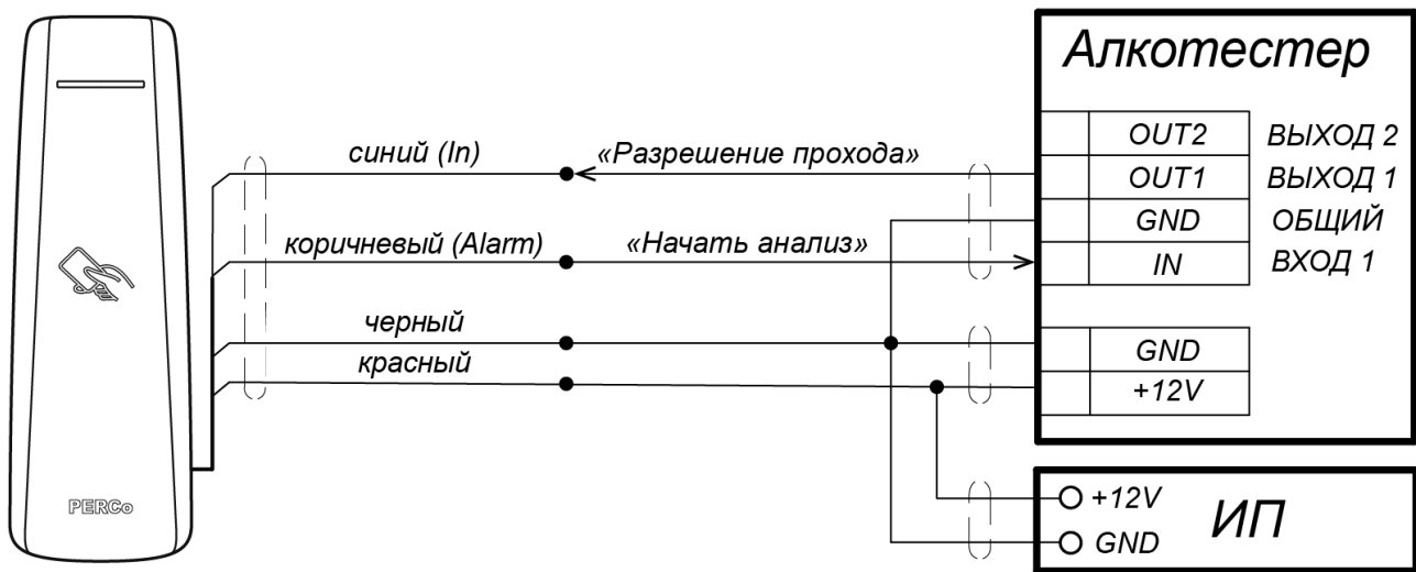
Рисунок 10. Схема подключения ВВУ на примере алкотестера
